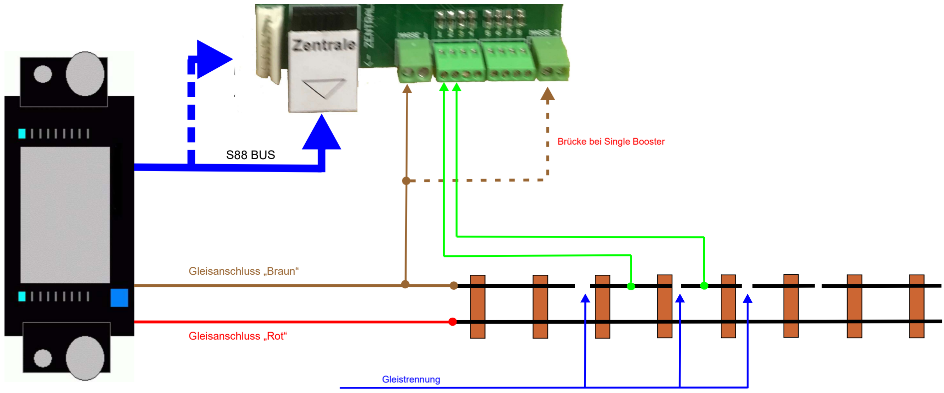
S88 Digital Zentrale
