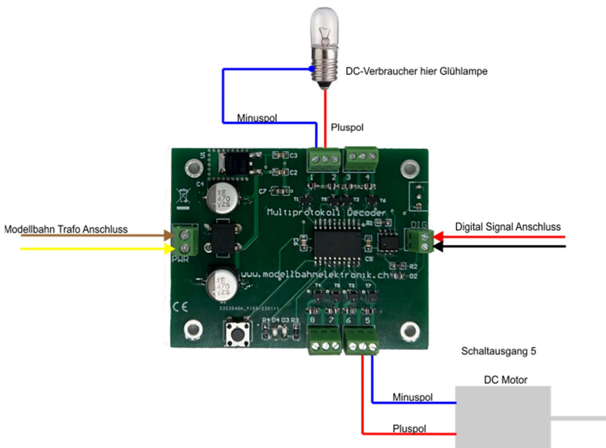
Skizze 2. Anschluss von Schaltartikel an den Decoder
