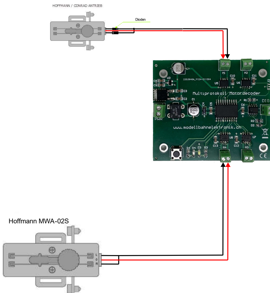
Skizze 2. Anschluss von Weichenmotoren an den Decoder
