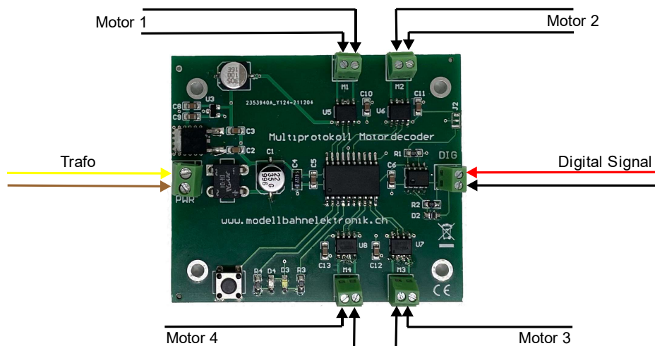
Skizze 1. Anschlüsse des Decoders
