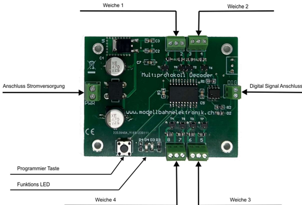
Skizze 1. Anschlüsse des Decoders
