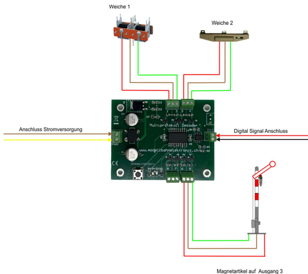
Skizze 2. Anschluss von Magnetartikel an den Decoder
